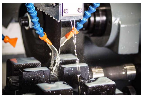
試材切断時の様子
