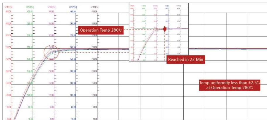
温度安定性 \pm 2.5^\circ\text{C} ( 280^\circ\text{C} )
