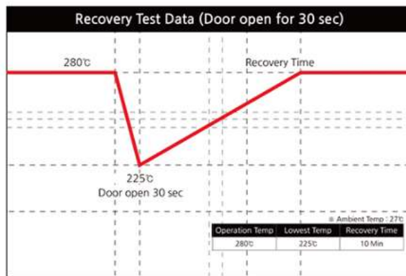
開扉後温度回復データ（赤線、開扉30秒後：10分）
