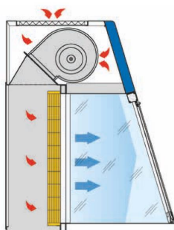
ベンチ内気流の模式図
