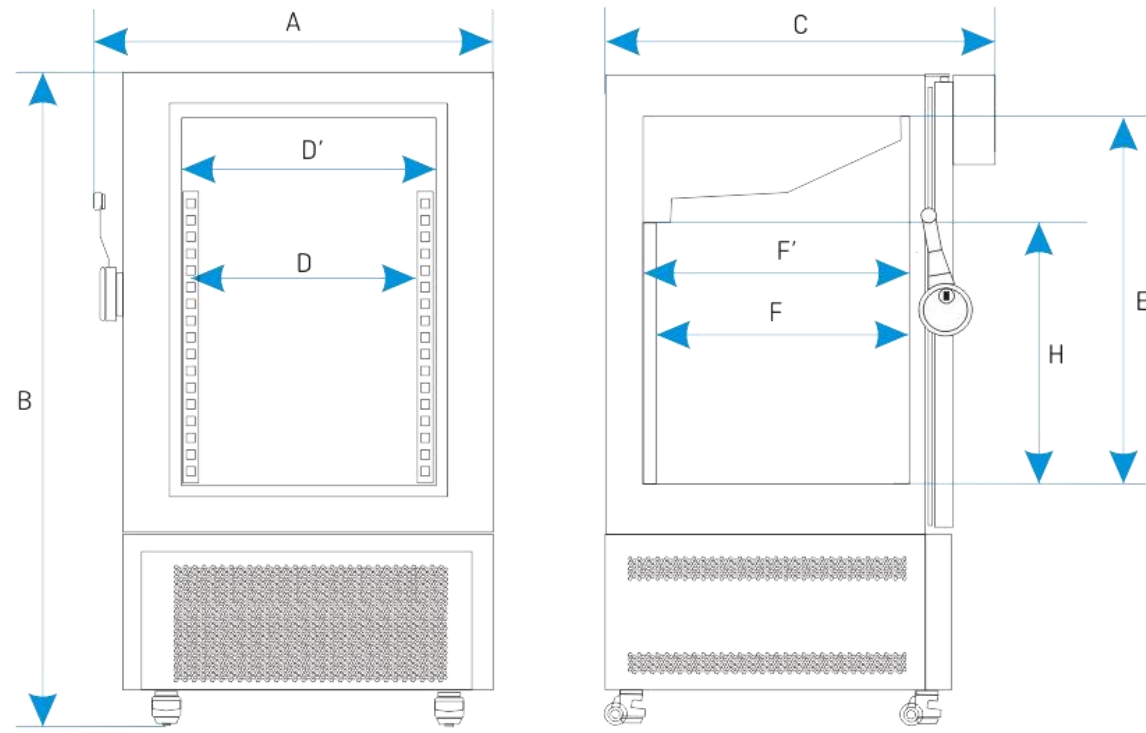
ZLW-T 200/300 モデル
