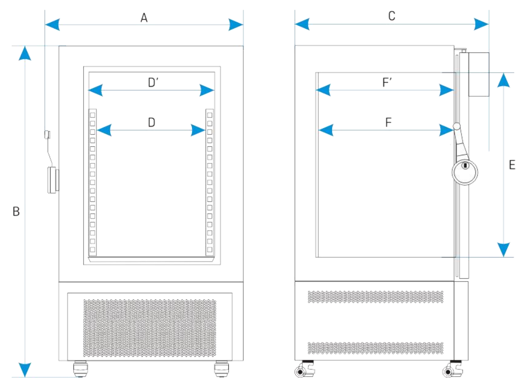
ZLN-T125/200/300 モデル
