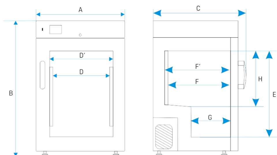
ZLN85 モデル
