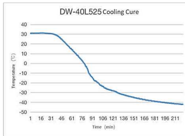
冷凍運転時の経時温度変化グラフ（参考※）
