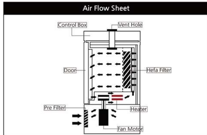
空気の流れ
