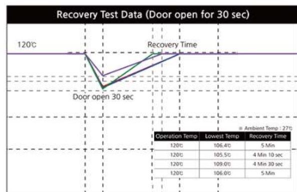
開扉後温度回復データ
