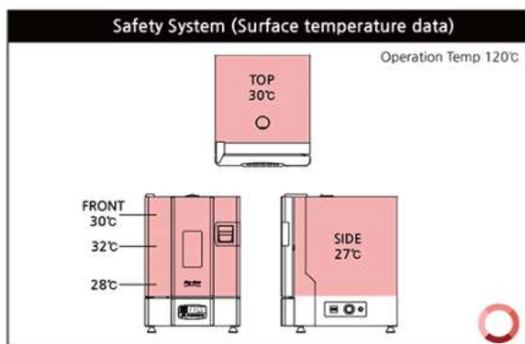
安全な表面温度 (120℃運転時)
